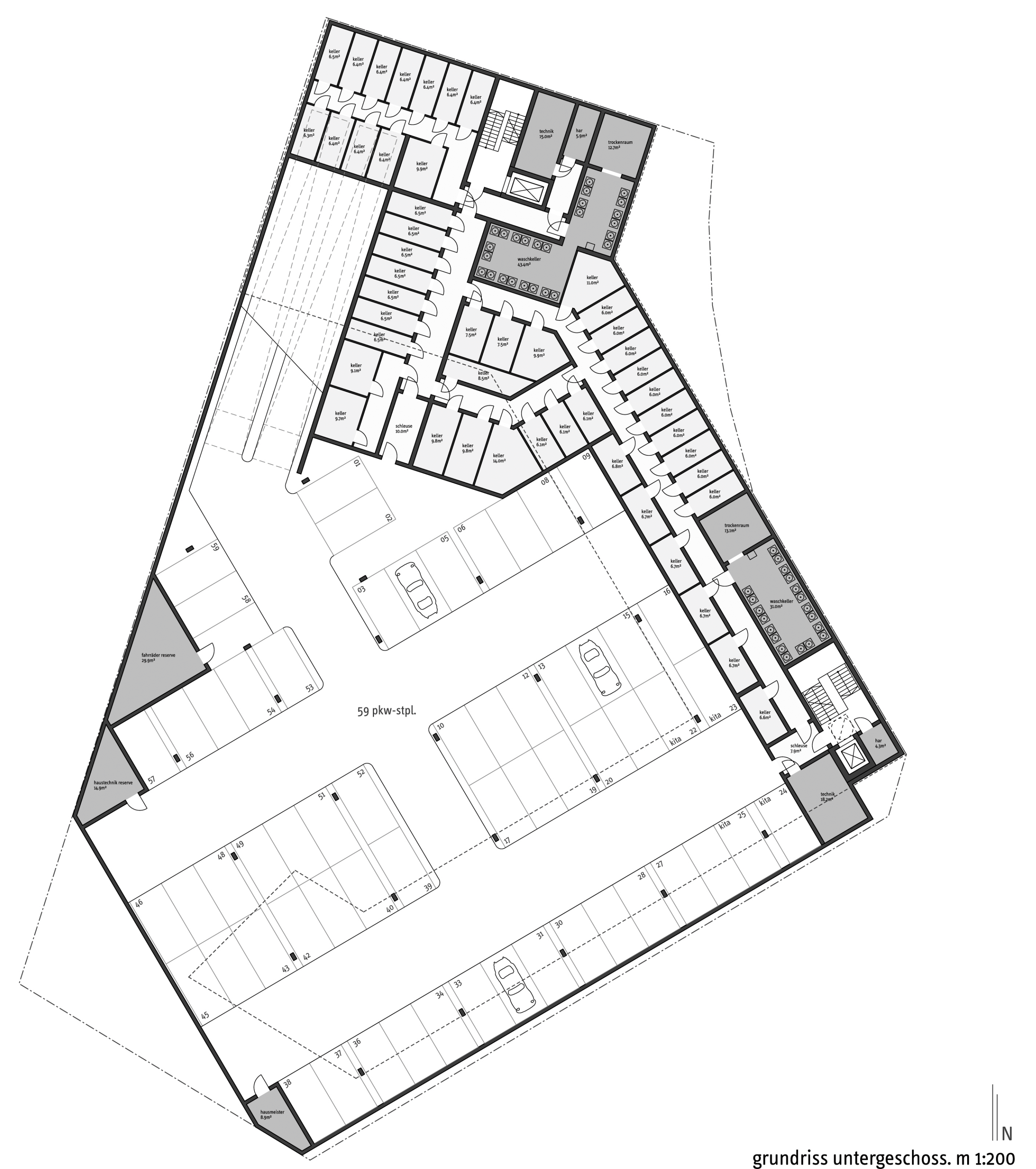
grundriss untergeschoss. m 1:200
